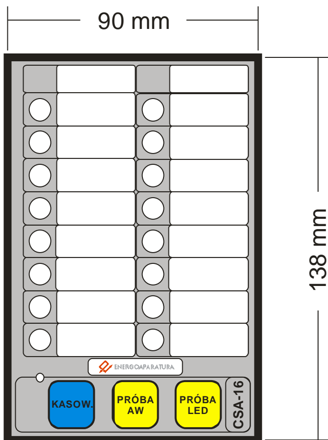
Rys 1. Rysunek wymiarowy- widok urządzenia od frontu
