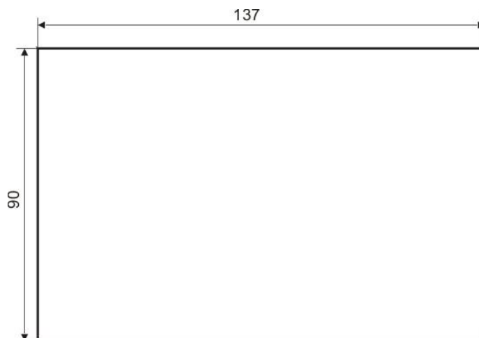
Rys 5. Otwór montażowy urządzenia CSA-16
