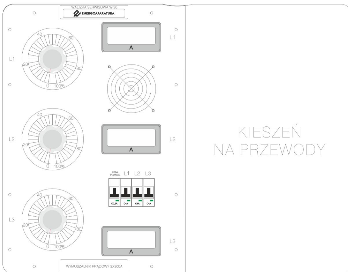
Rys. 1. Płyta frontowa walizki serwisowej W-30
