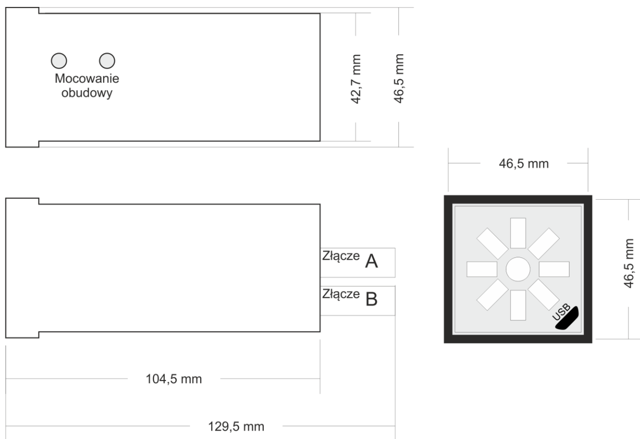
Rys. 3 Rysunek wymiarowy WPW-1
