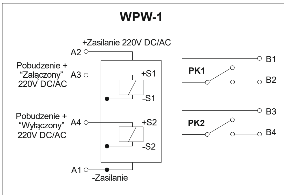
Rys. 2. WPW-1 rozkład wyprowadzeń.
