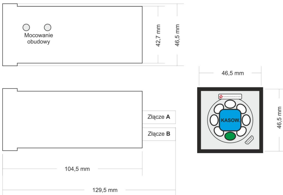
Rys. 2 Rysunek wymiarowy przełącznika PS-1 MINI
