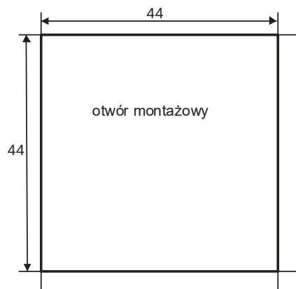
Rys. 3. Otwór montażowy dla przekaźnika PS-1 MINI
