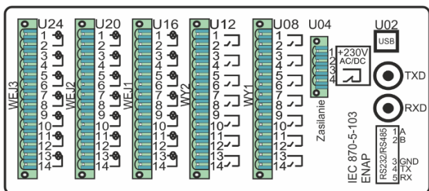
Rys. 2. Schemat funkcjonalny CSA-12
