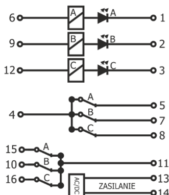
Rys. 2. Schemat funkcjonalny PKOW-1
