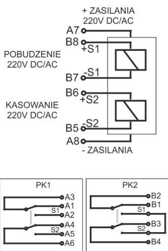
Rys. 2. Schemat funkcjonalny PS-1
