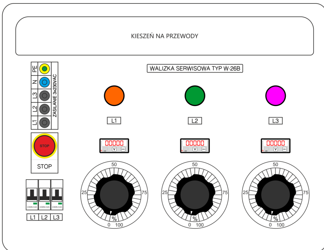
Rys.1 . Płyta frontowa walizki serwisowej W-26
