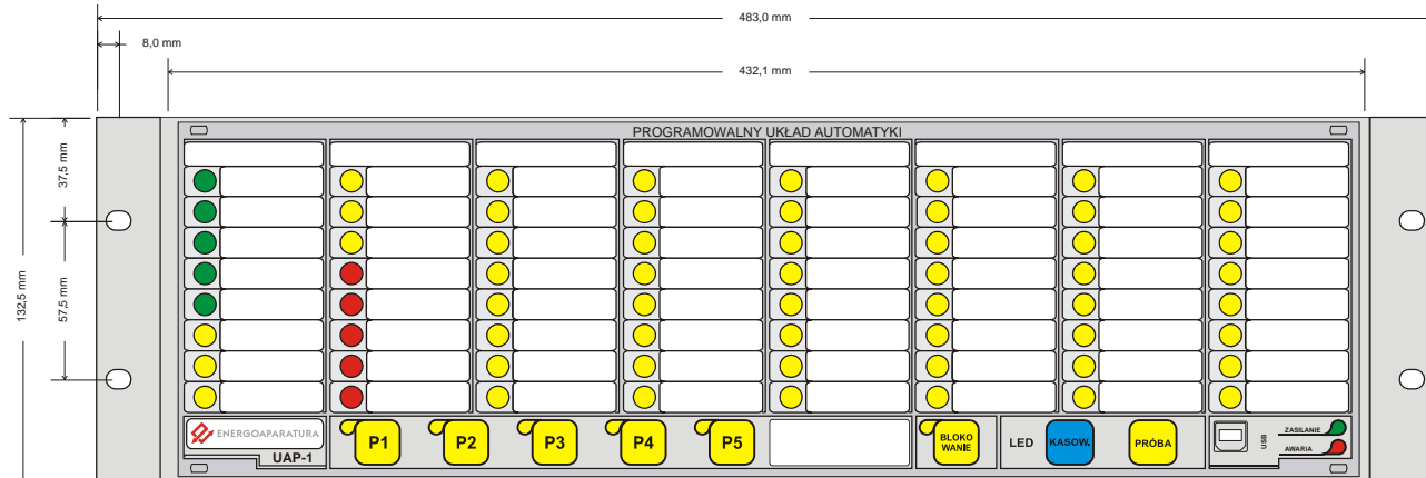
Rys. 1. Urządzenie UAP-1- widok od frontu.
