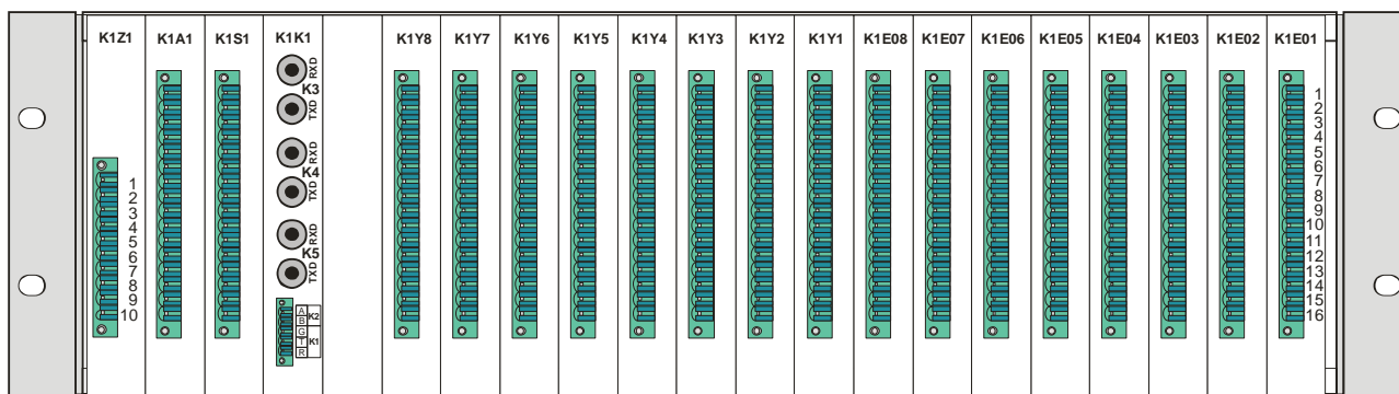
Rys.4. Urządzenie UAP-1 - widok od strony złącz - wersja z powieleniami.
