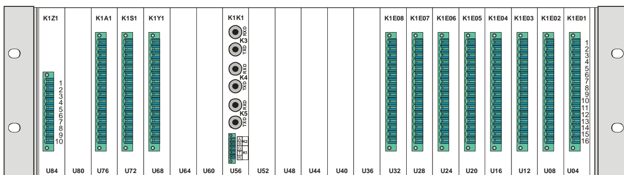
Rys. 2. Urządzenie UAP-1 - widok od strony złączy (wersja podstawowa).
