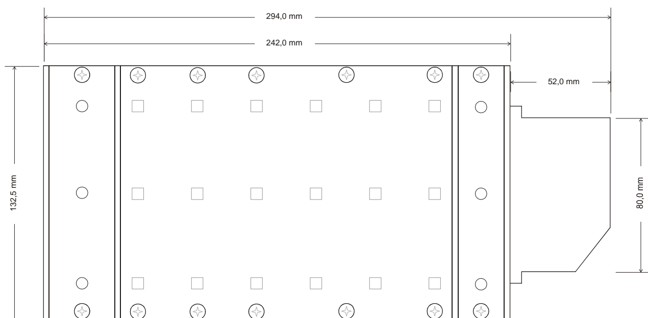
Rys. 3. Urządzenie UAP-1 - widok z boku.
